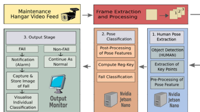
Fig. 2. Proposta da arquitetura do sistema de detecção de quedas, retirado de [15]
